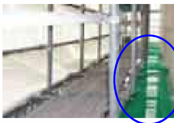
비계와 벽체 사이 추락보호망
